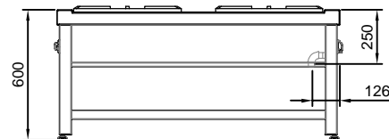
CONEXÃO DE GÁS 1/2" NPT VISTA LATERAL
