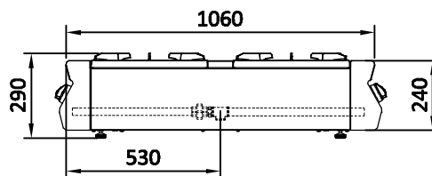
CONEXÃO DE GÁS 3/4" BSP VISTA LATERAL
