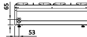
CONEXÃO DE GÁS 3/4" BSP VISTA TRASEIRA
