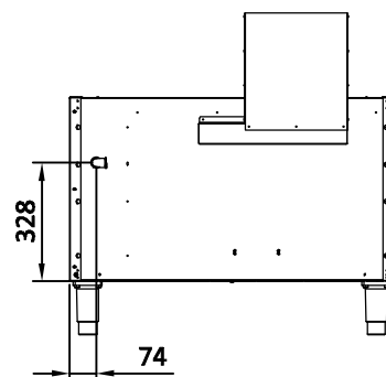
CONEXÃO DE GÁS 1/2" BSP VISTA TRASEIRA
