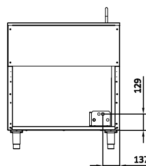
CONEXÃO DE GÁS 1/2" NPT VISTA TRASEIRA
