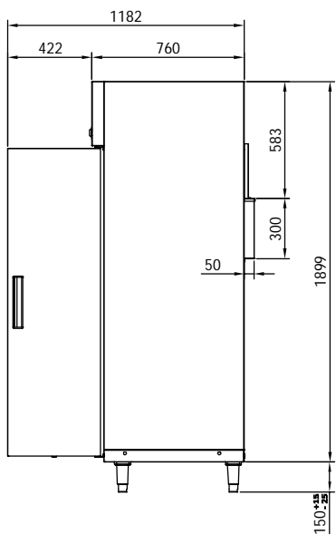
VISTA LATERAL
