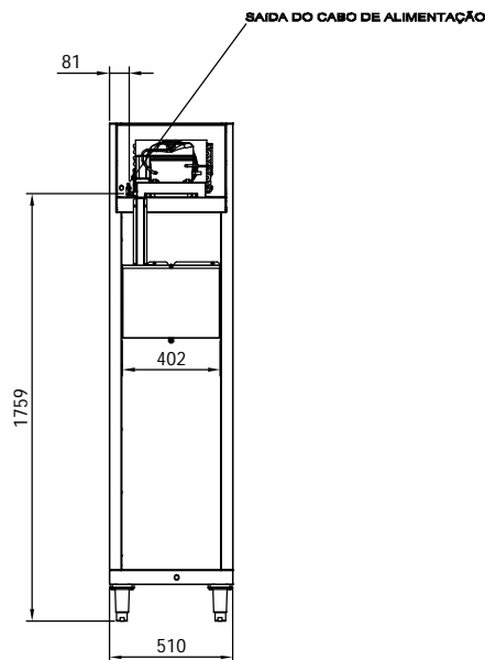
VISTA TRASEIRA
