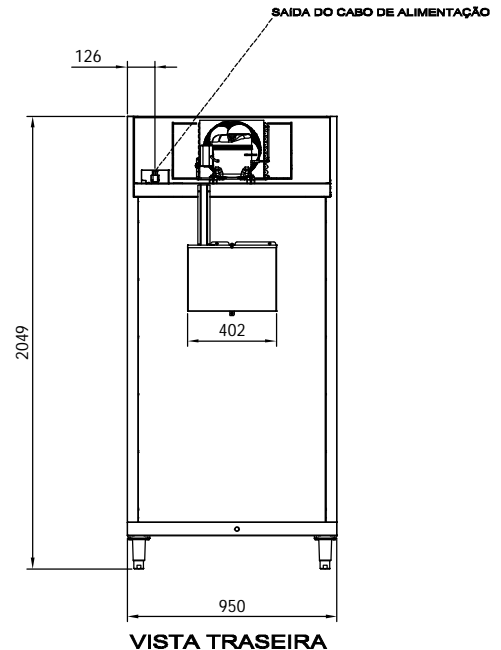
VISTA TRASEIRA
