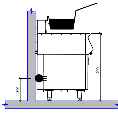
VISTA LATERAL
