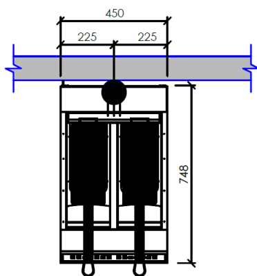
VISTA SUPERIOR
